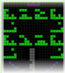
Нуклеотиди
